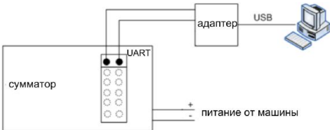
Рисунок 3. Общая схема электрических подключений Сумматора ДУТ
