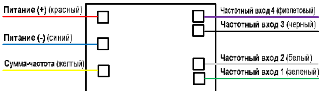
Рисунок 2. Назначения и цвета проводов Сумматора Ч
